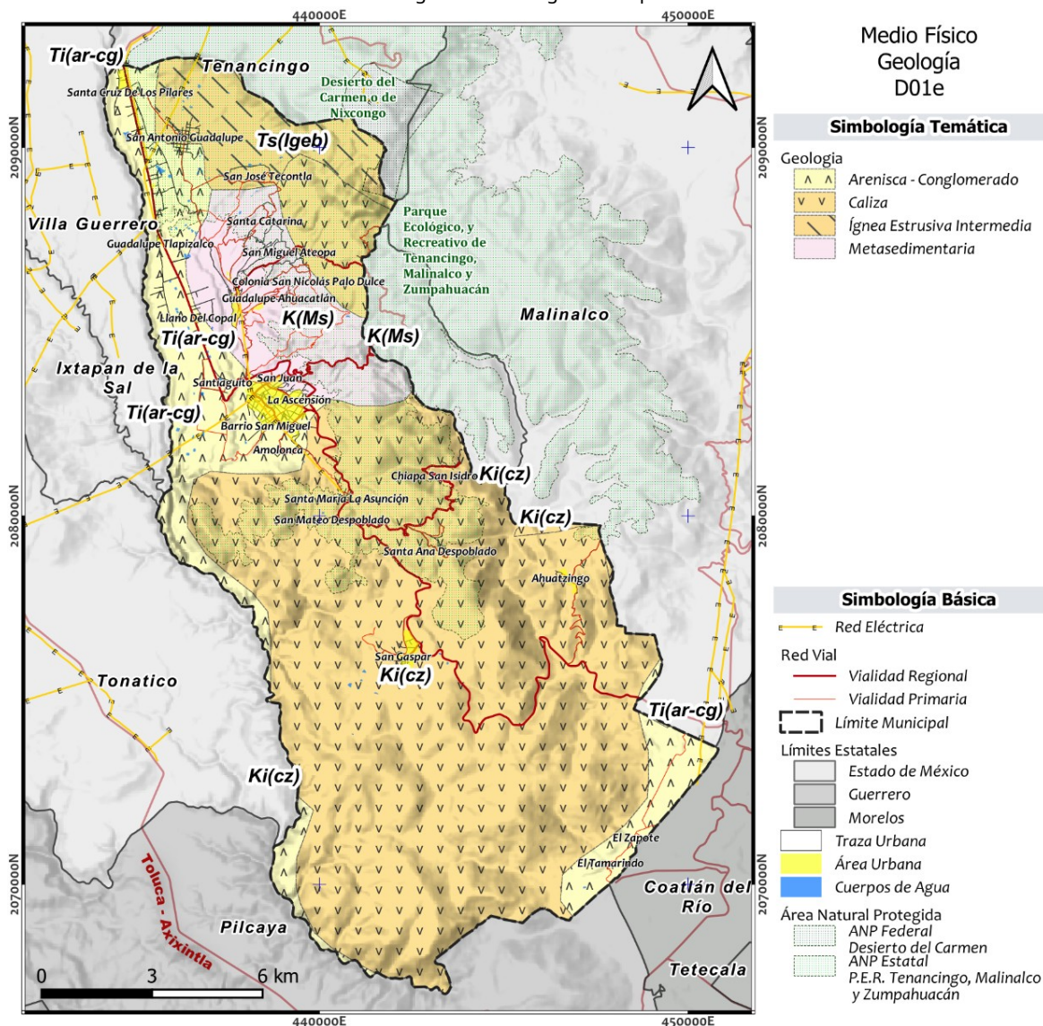
Figura 17. Geología municipal.
