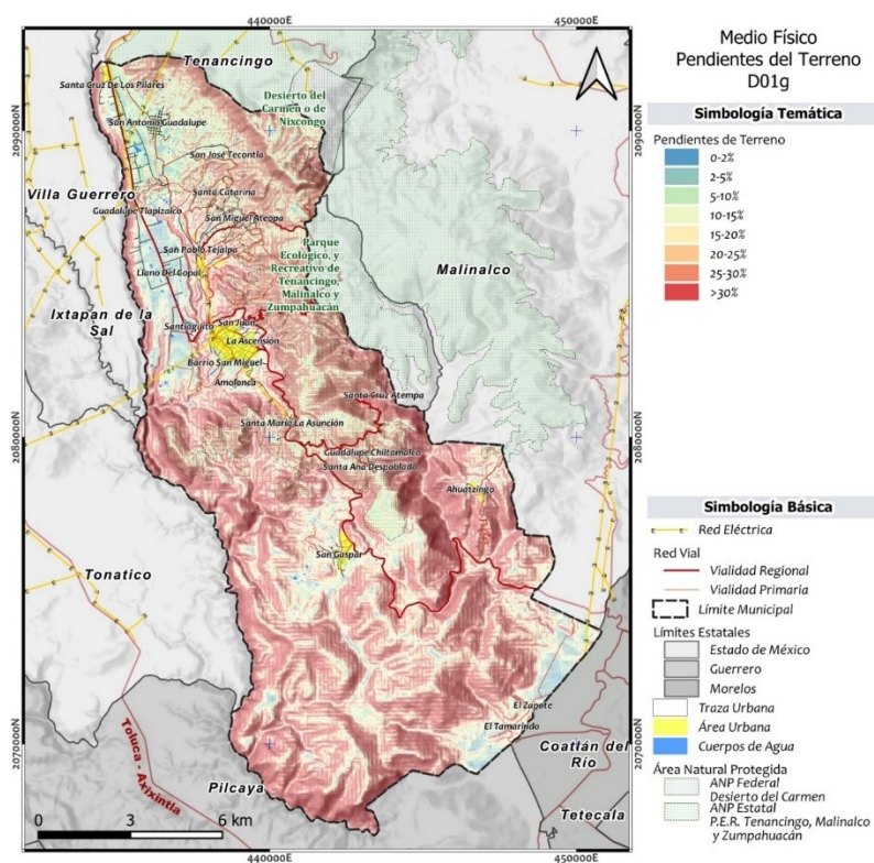
Figura 15. Pendientes de terreno en el municipio de Zumpahuacán.
