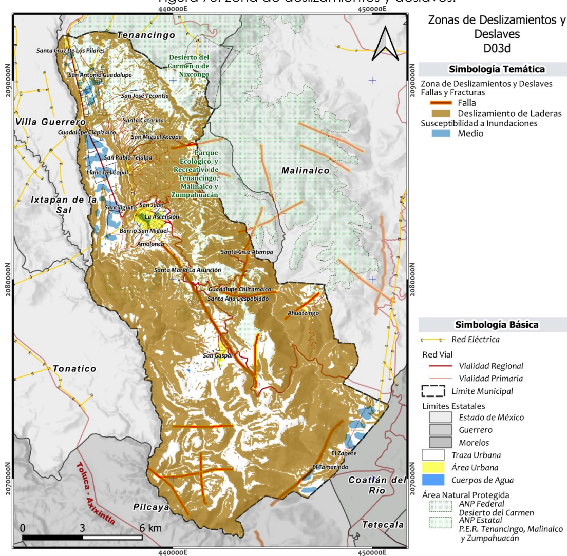
Figura 73. Zona de deslizamientos y deslaves.
